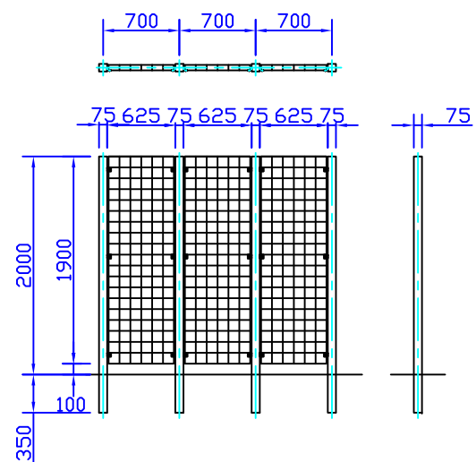
W600×D50×H1900(縦)
