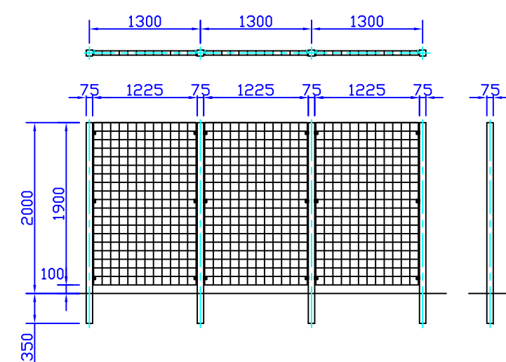
W1200×D50×H1900(縦)
