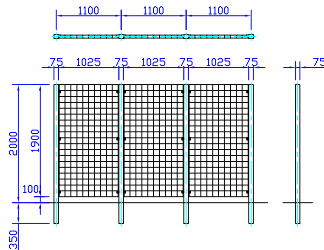
W1000×D50×H1900(縦)
